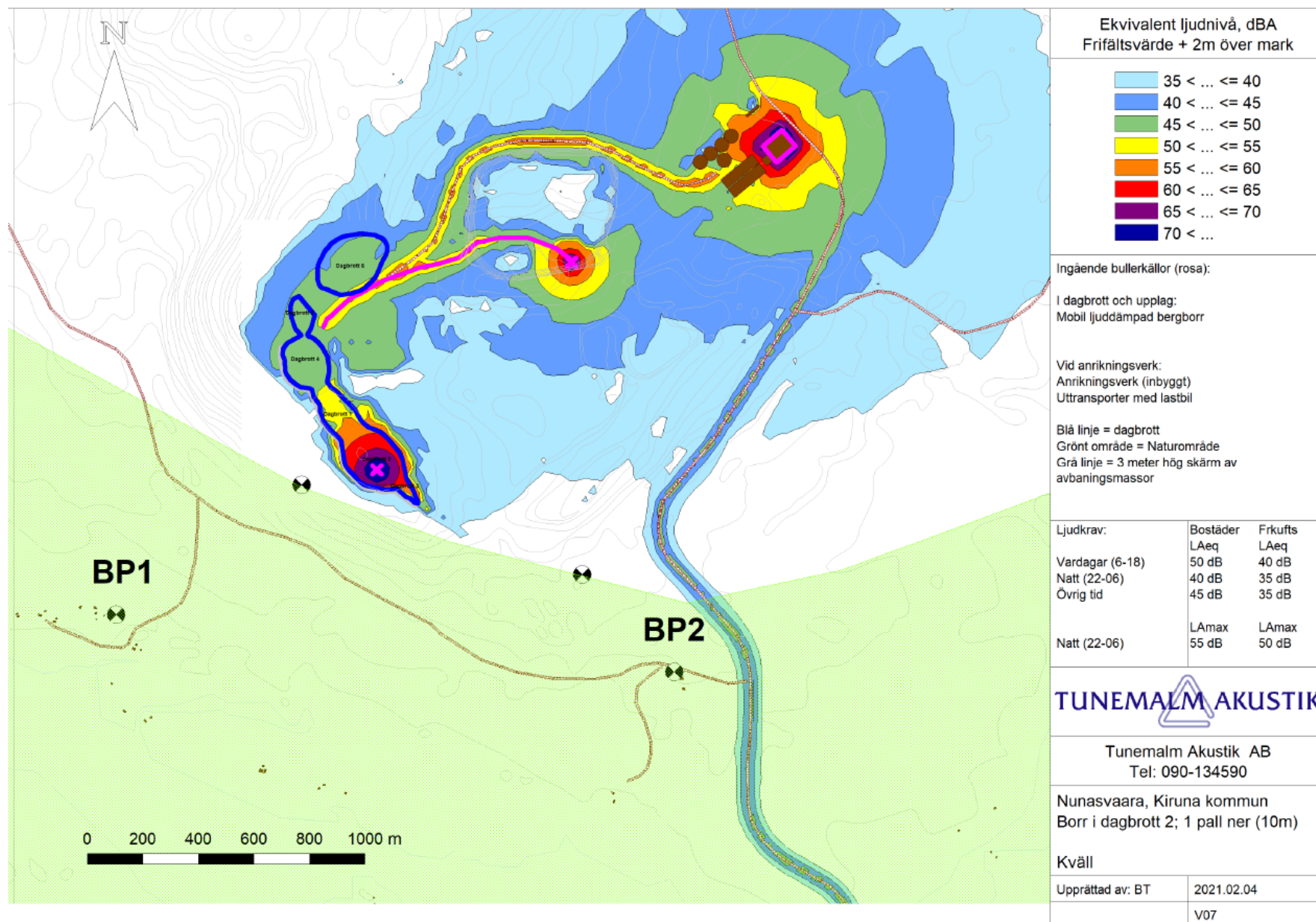
Figur 8: Dagbrott 2, en pall ner 10 m, efter 1 års produktion. Ljudutbredning med 3 m bullervall, se grålinje, och luddämpad borrhög. Den ljusgröna ytan är riksintresse friluftsliv Torne älv.
