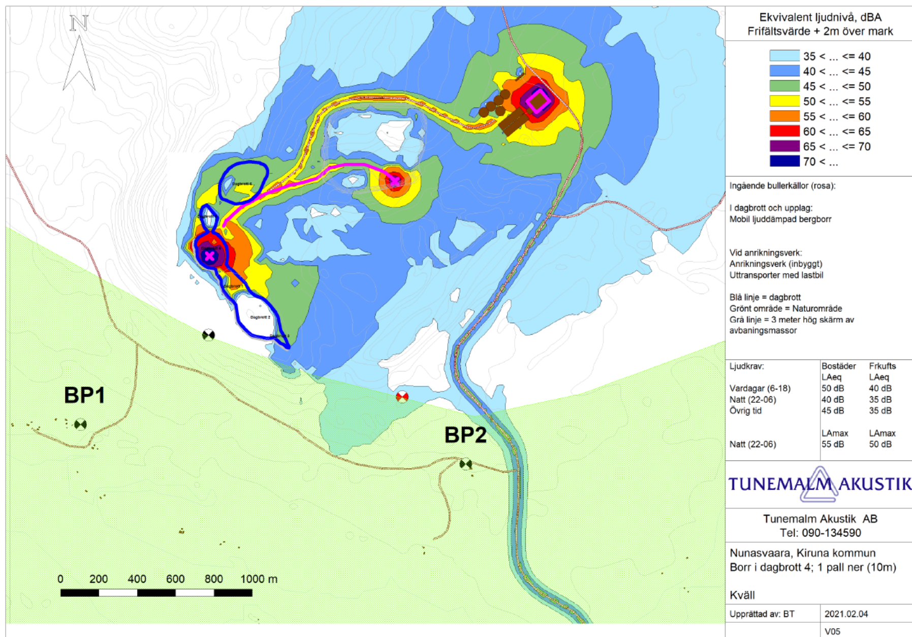
Figur 10: Dagbrott 4 en pall ner 10 m, efter 1 års produktion. Ljudutbredning med 3 m bullervall, se grålinje, och ljuddämpad borrhög. Den ljusgröna ytan är riksintresse friluftsliv Torne älv.
