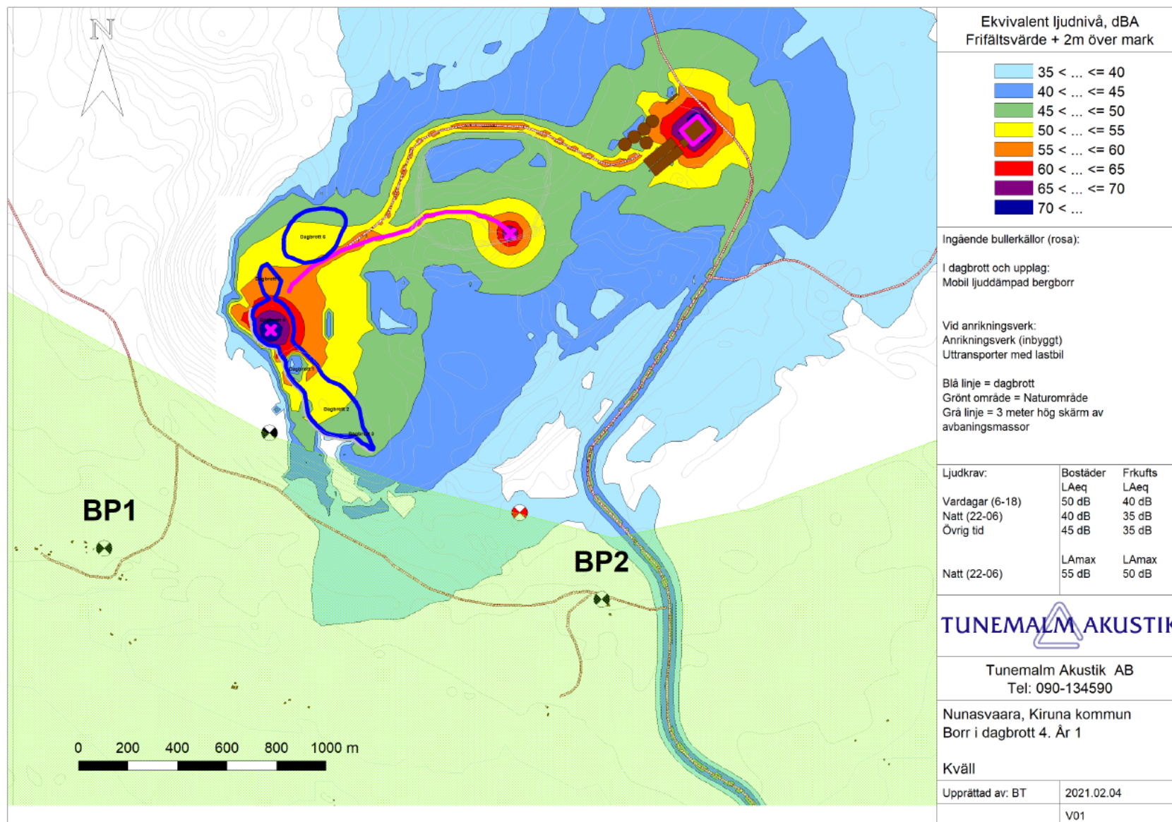
Figur 6: Dagbrott 4 år 1, ljudutbredning med 3 m bullervall, se grålinje, och luddämpad borrhigg. Den ljusgröna ytan är riksintresse friluftsliv Torne älv.
