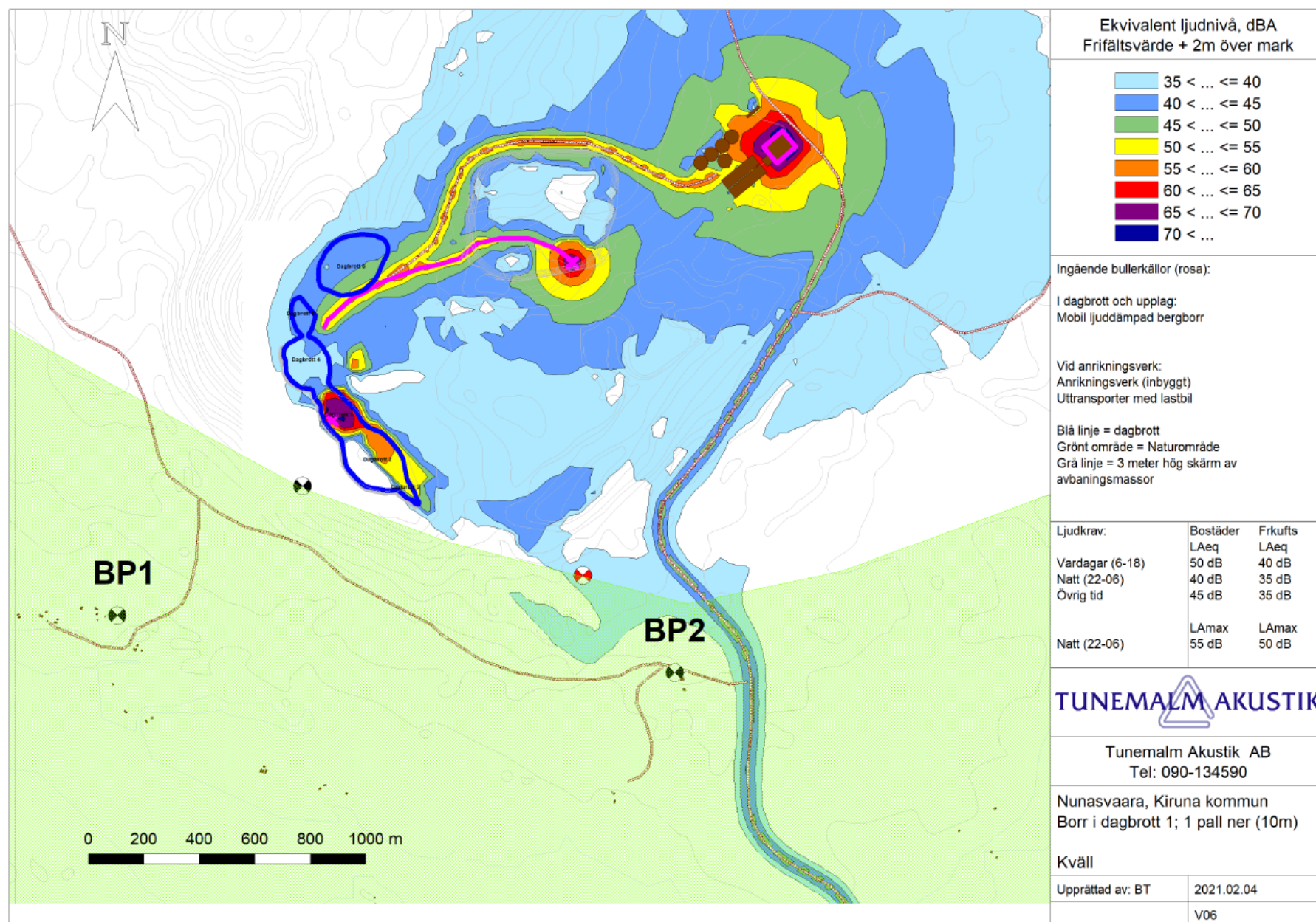
Figur 9: Dagbrott 1, en pall ner 10 m, efter 1 års produktion. Ljudutbredning med 3 m bullervall, se grålinje, och ljuddämpad borrhög. Den ljusgröna ytan är riksintresse friluftsliv Torne älv.
