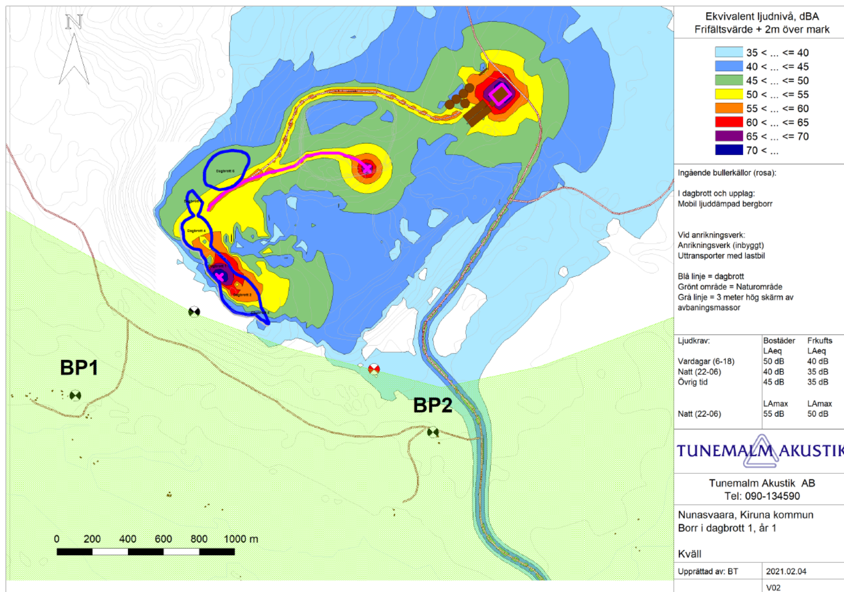
Figur 7: Dagbrott 1 år 1, ljudutbredning med 3 m bullervall, se grålinje, och luddämpad borrhög. Den ljusgröna ytan är riksintresse friluftsliv Torne älv.
